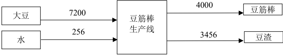
图 2-1 物料平衡图 单位：t/a
